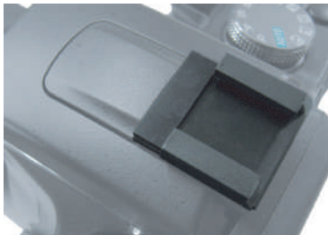
ソニーα用変換シュー UNX-8519 085191 ● ￥648-(税別) サイズ:H9×W22×D24mm、重量:約1.5gシンクロ(同調)機能はありません。 ソニーマルチインターフェースシュータイプの製品には取り付けはできません。
